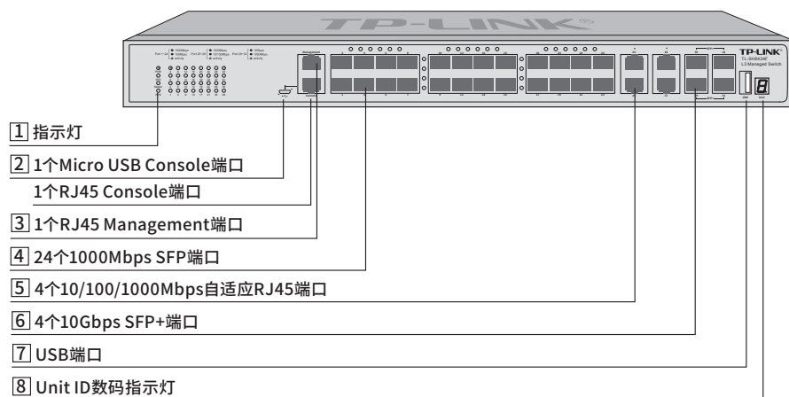
图1-2 TL-SH8434F前面板示意图
