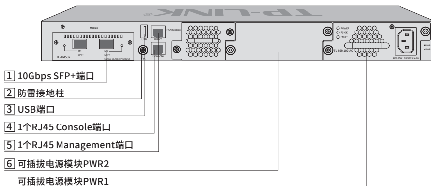
图1-6 TL-SH8452后面板示意图
