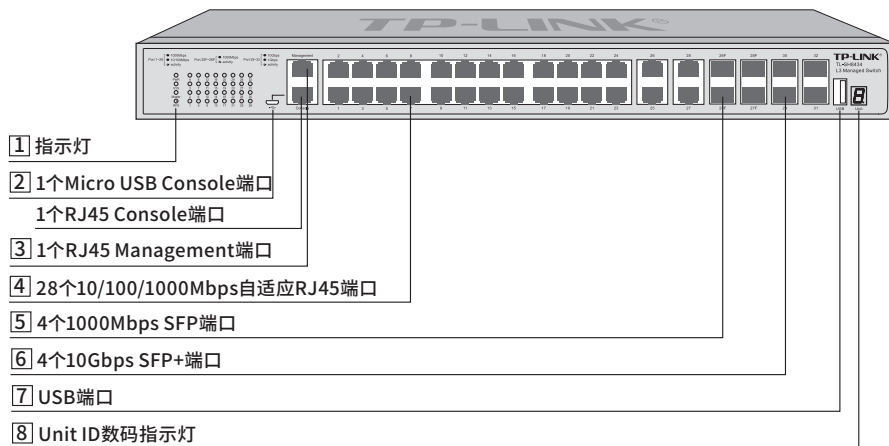
图1-1 TL-SH8434前面板示意图
