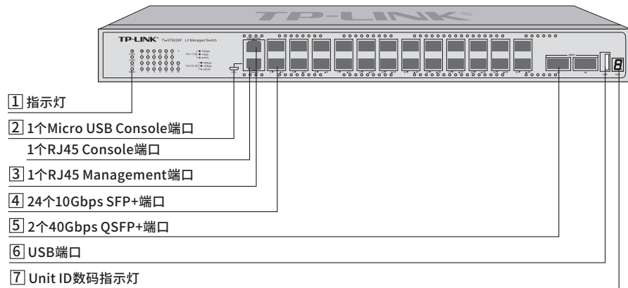
图1-4 TL-ST8226F前面板示意图
