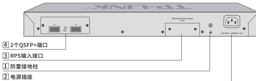
图1-5 TL-SH8434后面板示意图
