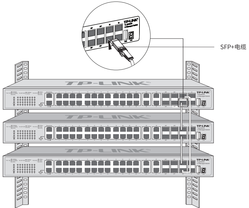
图2-4 使用SFP+端口建立堆叠示意图
