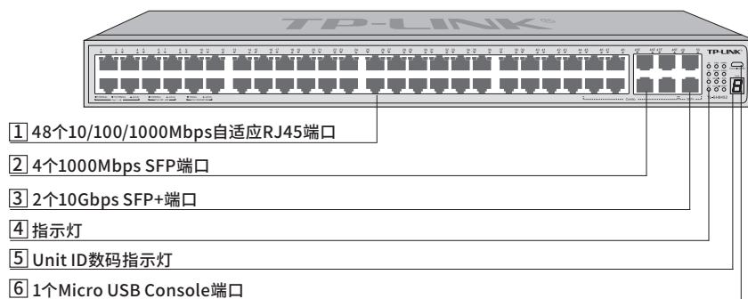
图1-3 TL-SH8452前面板示意图
