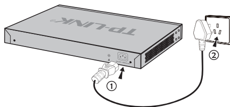
图3-5 电源线连接示意图
