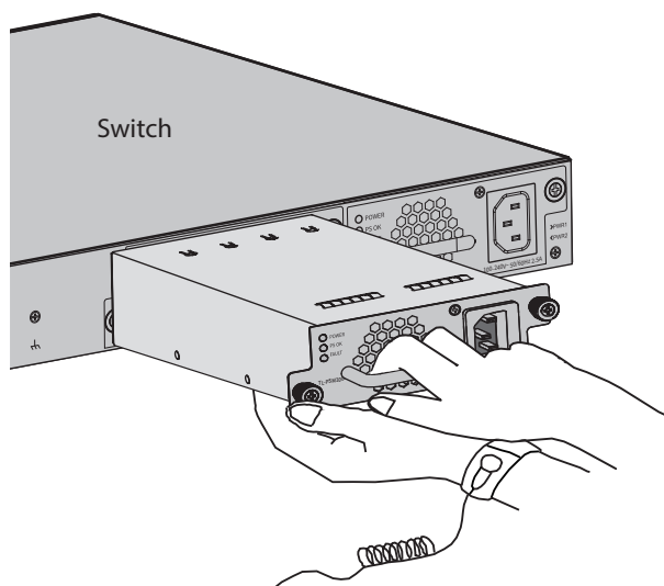
图3-7 安装电源模块示意图
